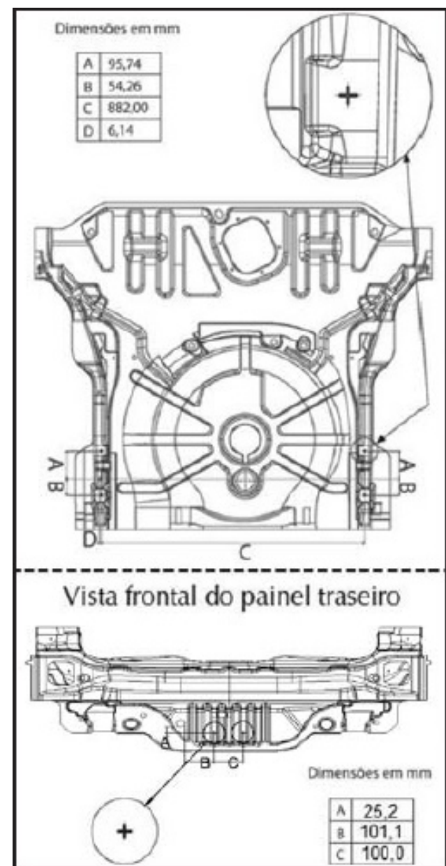
Vista superior do assoalho traseiro
